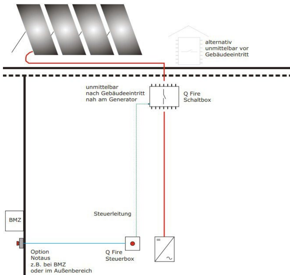
Abbildung 1: Übersicht Montageposition
