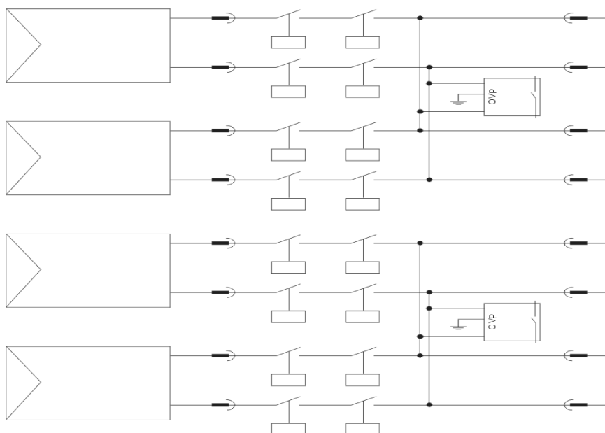
Abbildung 17: Verschaltung Strings und Überspannungsschutz SPD
