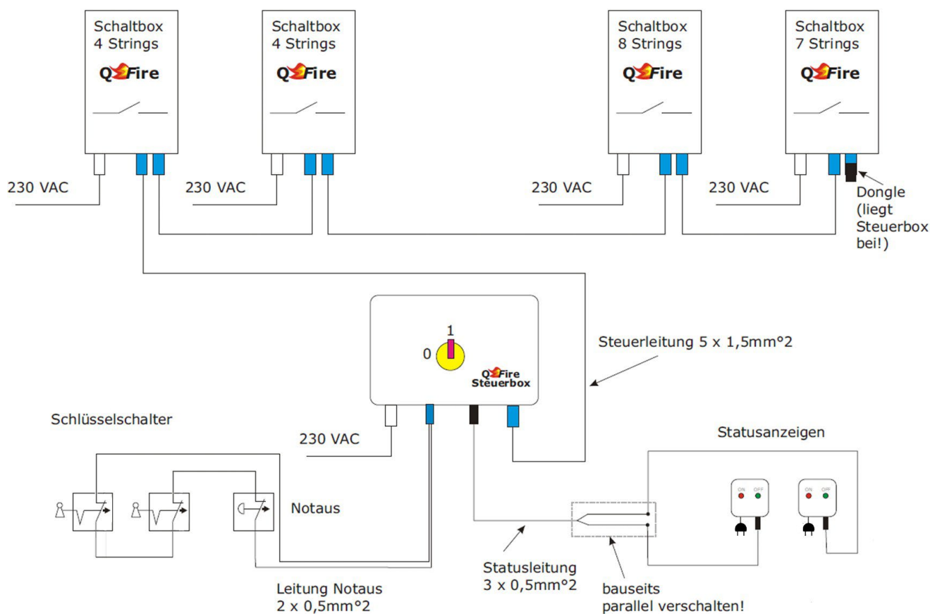
Abbildung 2: Layoutbeispiel
