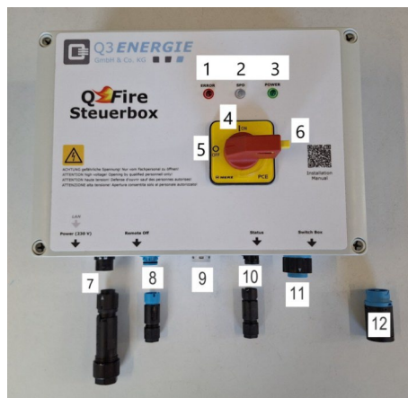
Abbildung 5: Steuerbox
