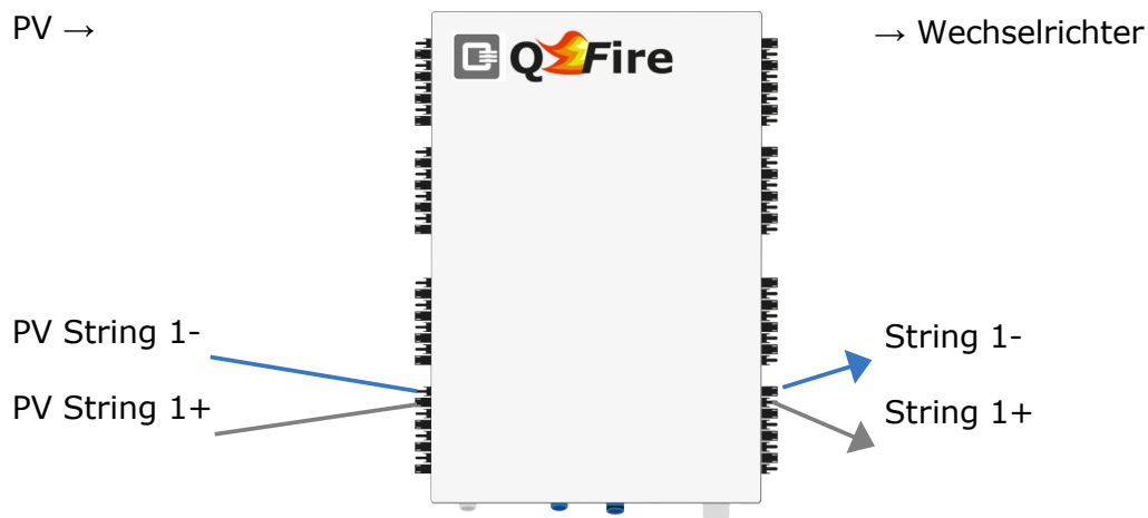
Abbildung 16: Anschlüsse Schaltbox
