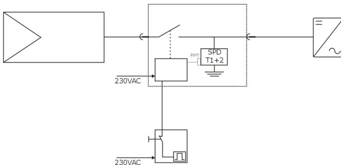
Abbildung 14: Schaltplan QFire
