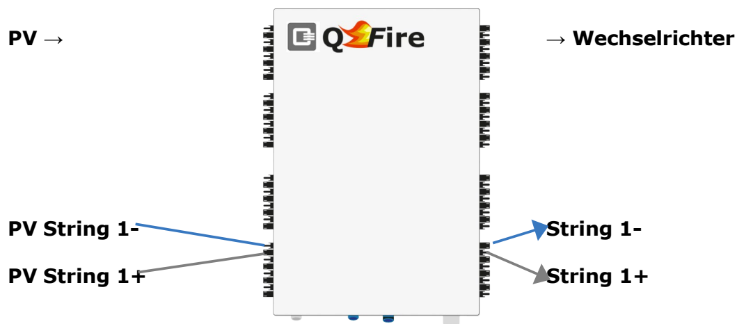
Abbildung 16: Anschlüsse Schaltbox
