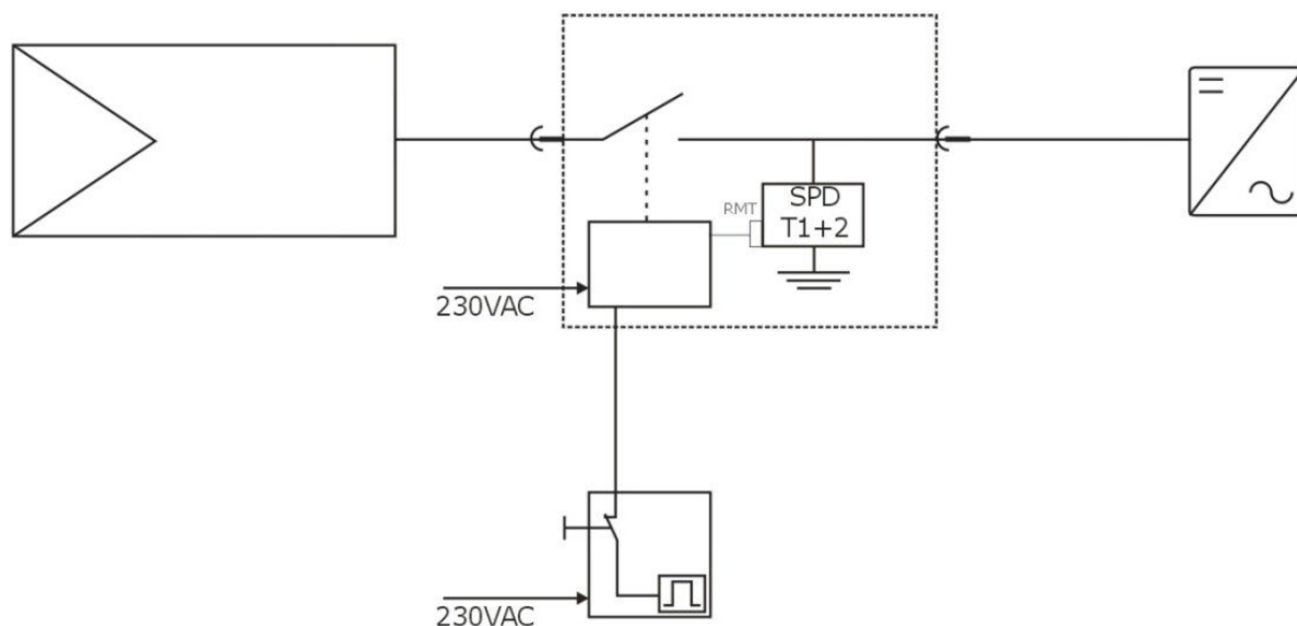
Abbildung 14: Schaltplan QFire
