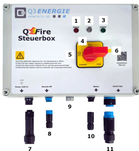
Abbildung 5: Steuerbox
