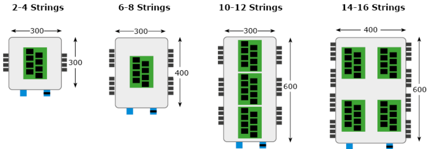
Abbildung 11: Abmessungen der Schaltbox-Varianten in mm
