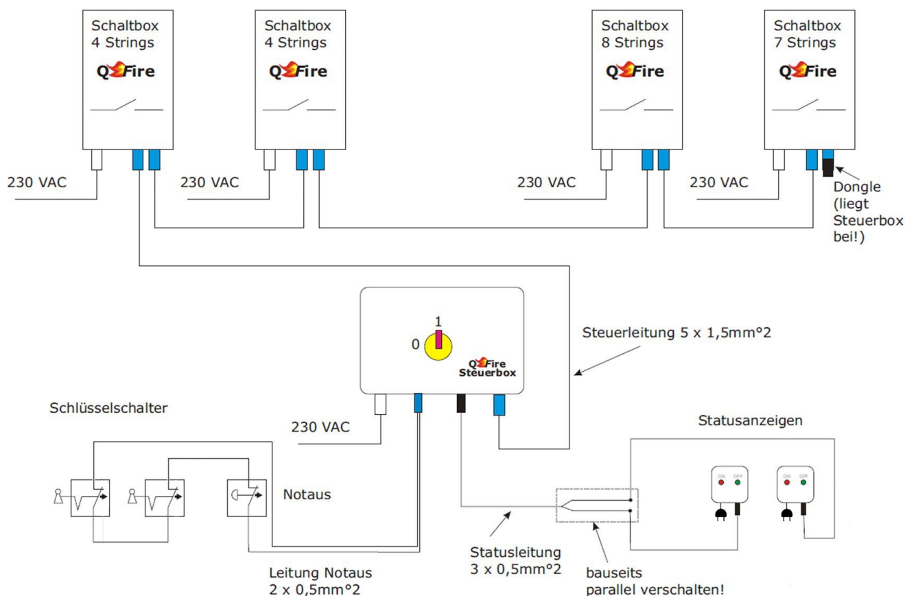
Abbildung 2: Layoutbeispiel
