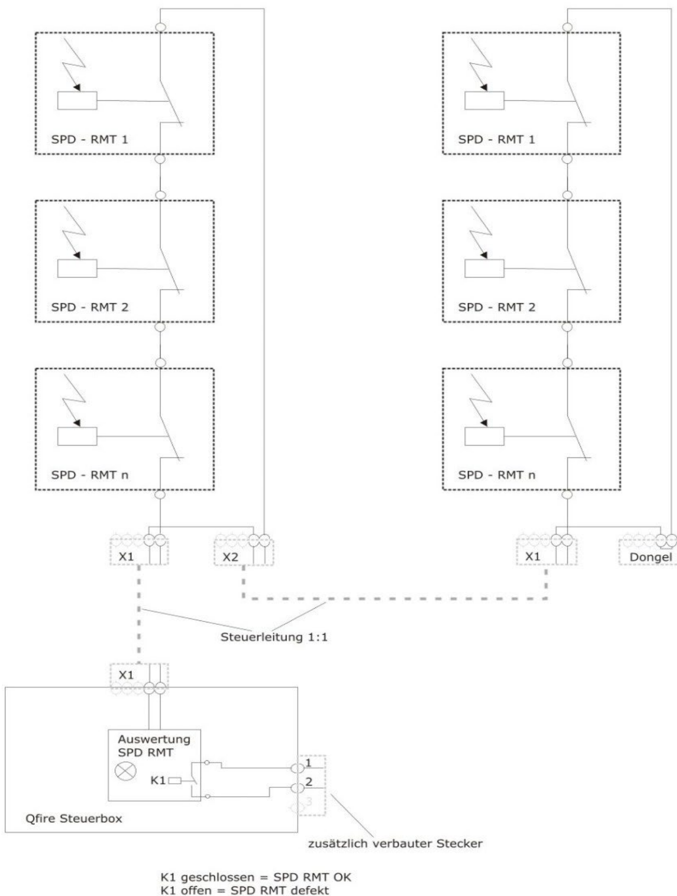
Abbildung 19: Schaltbild SPD RMT
