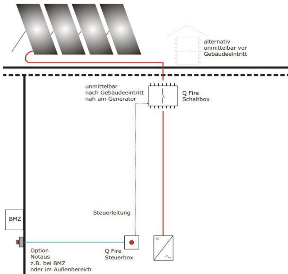
Abbildung 1: Übersicht Montageposition
