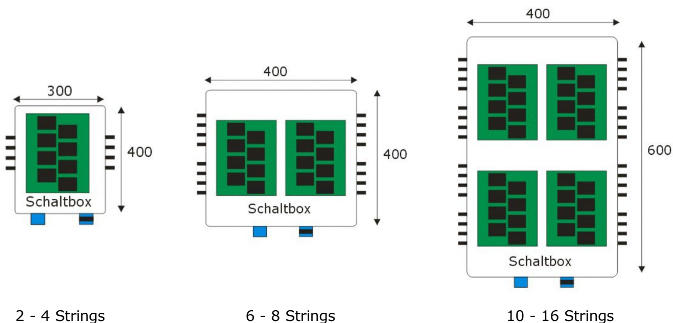
Abbildung 11: Abmessungen der Schaltbox-Varianten in mm
