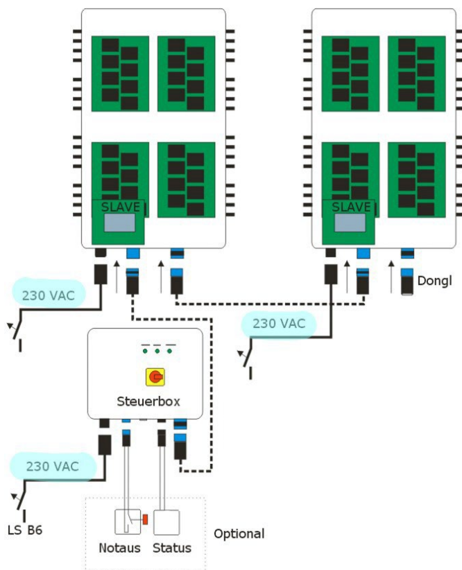
Abbildung 15: Steuerleitungen Anschluss Schaltbox(en)
